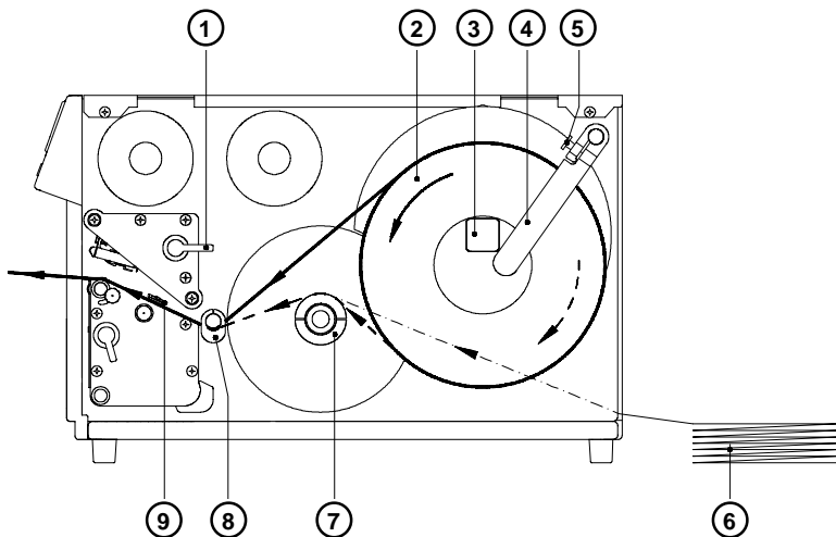
Bild 6 b Einlegen der Etiketten Apollo 2/3
