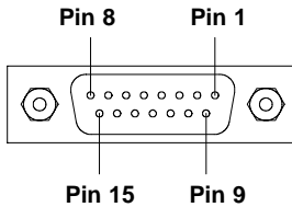
Bild B-7 Peripherieanschlußbuchse
