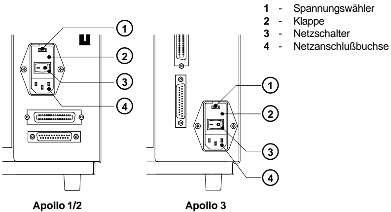
Bild 5 a Netzmodul (Detailansicht Druckerrückseite)
