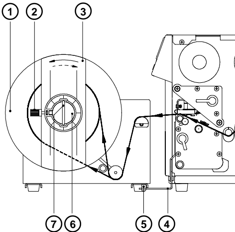
Bild 13 f Aufwickeln direkt auf die Wickelachse
