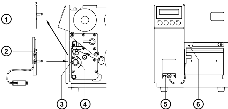
Bild 13 m Montage des Spendesensors
