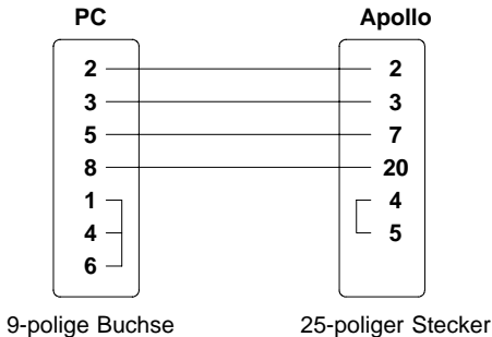
Bild B-3 Schnittstellenkabel mit 9-poligem Computeranschluß für RS-232 mit Protokoll " ---" bzw. "XON/XOFF"
