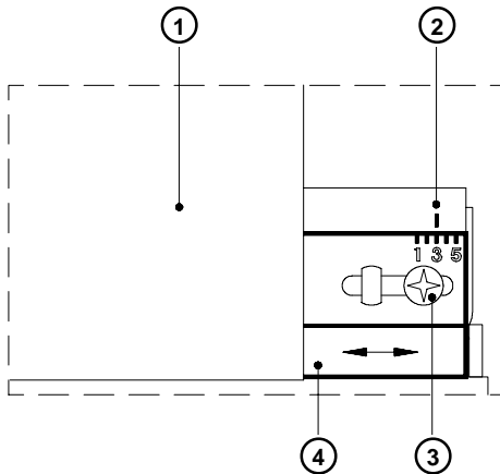
Bild 7 c Justage des Transferbandlaufes
