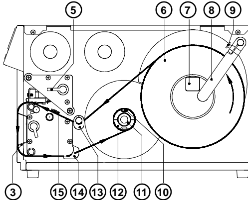
Bild 13 | Einlegen der Etiketten
