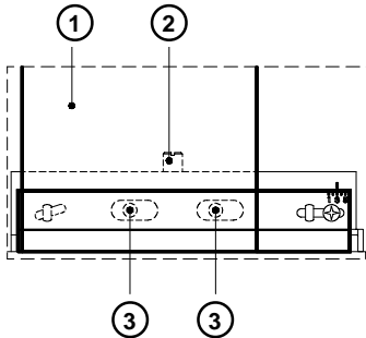
Bild D Druckkopfjustage
