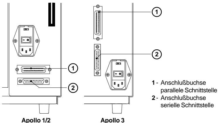
Bild 5 b Schnittstellenanschlüsse (Detailsicht Druckerrückseite)
