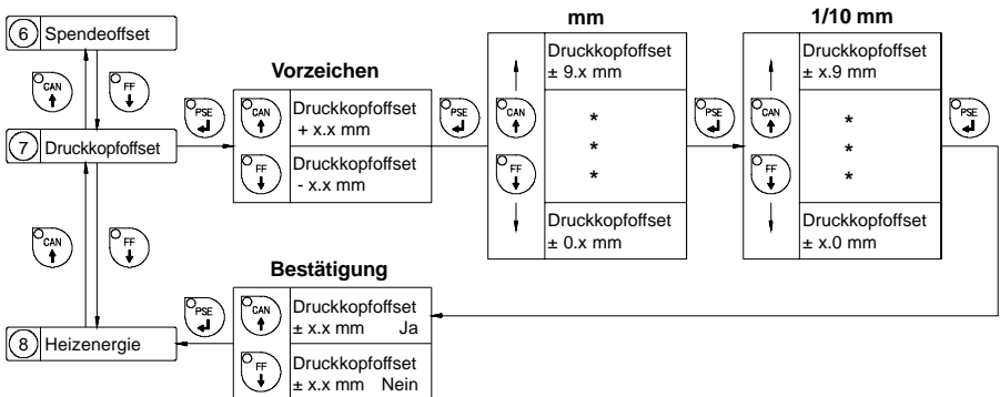
Bild 9 h Einstellung des Parameters "Druckkopffset"
