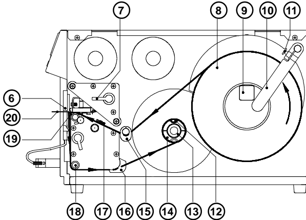
Bild 13 n Einlegen der Etiketten
