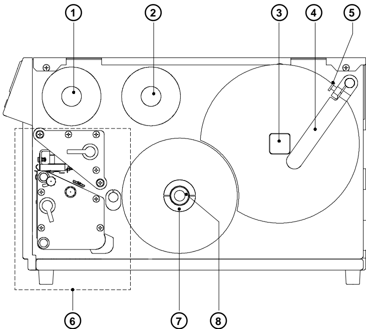
Bild 4 d Seitenansicht Apollo 2/3 (bei offenem Deckel)
