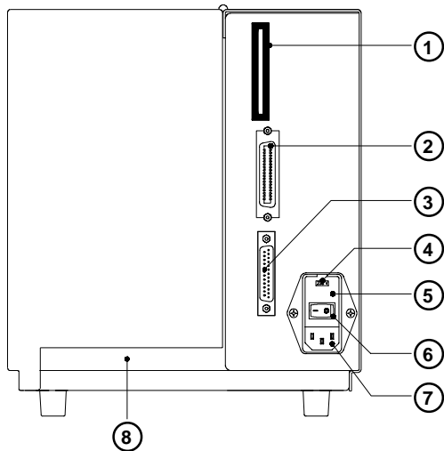
Bild 4 g Rückansicht Apollo 3
