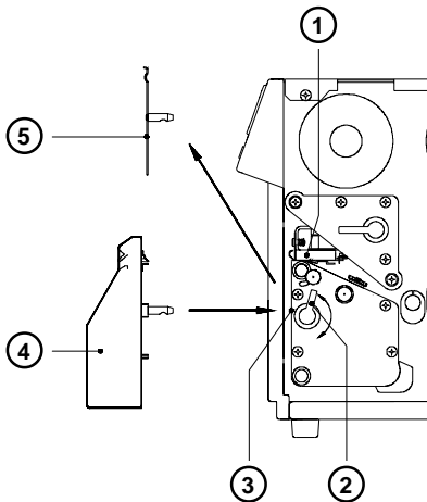
Bild 13 h Mechanische Kopplung des Schneidmessers
