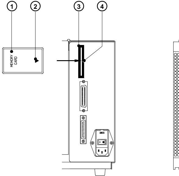
Bild 13 p Installation der Speicherkarte
