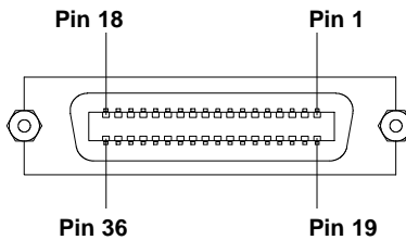
Bild B-6 Centronics-Buchse (Druckerrückseite)
