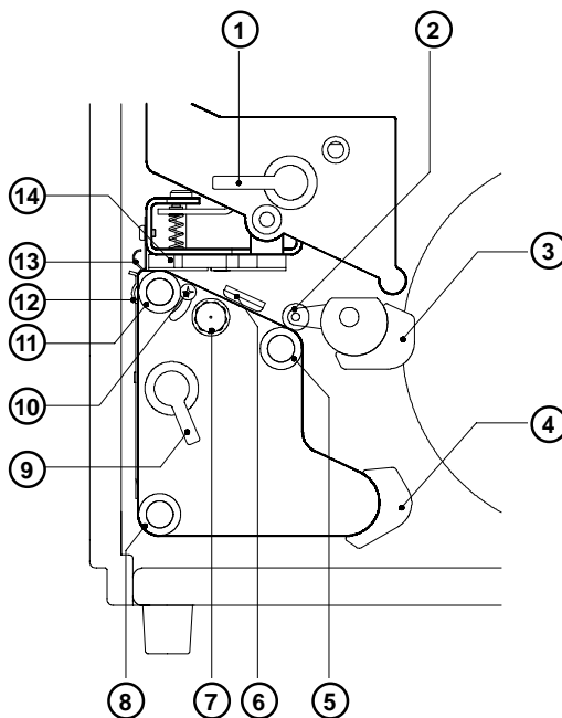
Bild 4 c Detailansicht Druckmechanik Apollo 1
