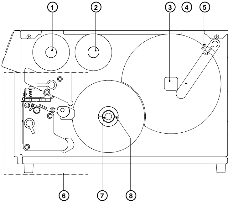
Bild4 b Seitenansicht Apollo 1 (bei offenem Deckel)
