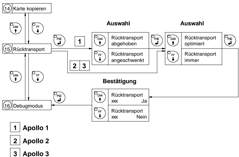
Bild 9 q Einstellung des Parameters "Rücktransport"
