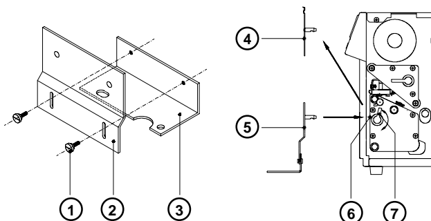
Bild 13 b Montage des Druckeradapters
