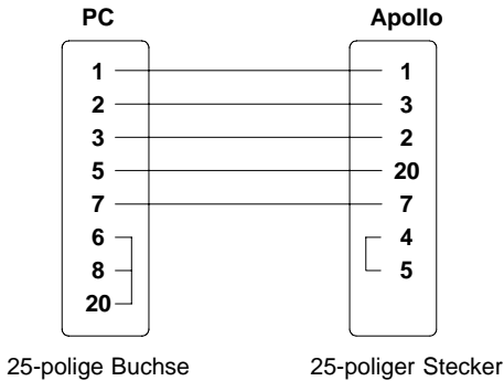
Bild B-2 Schnittstellenkabel mit 25-poligem Computeranschluß für RS-232 mit Protokoll " ---" bzw. "XON/XOFF"
