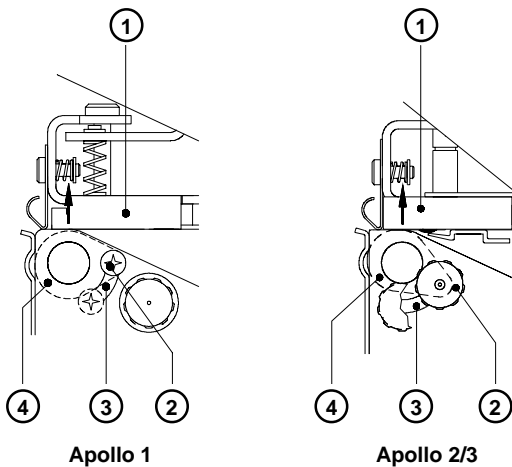
Bild 7 b Justage der Druckkopfabstützung
