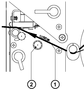
Bild 7 a Justage der Etikettenlichtschranke
