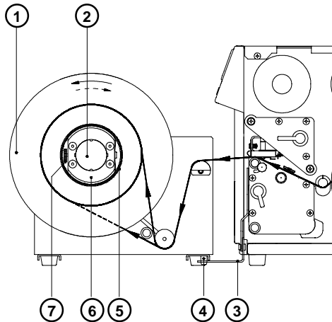
Bild 13 g Aufwickeln auf 75-mm-Papphülse (Darstellung ohne Flansch)
