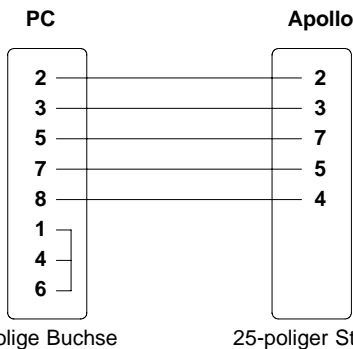
Bild B-5 Schnittstellenkabel mit 9-poligem Computeranschluß für RS-232 mit Protokoll "RTS/CTS" bzw. "XON/XOFF"
