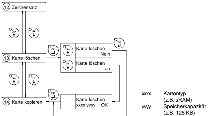
Bild 9 o Löschen/Formatieren einer Speicherkarte
