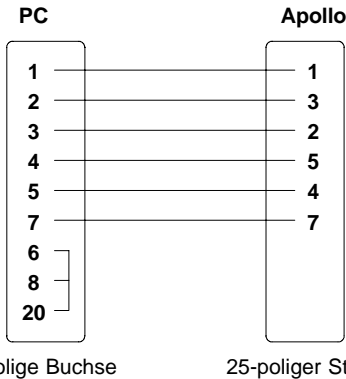
Bild B-4 Schnittstellenkabel mit 25-poligem Computeranschluß für RS-232 mit Protokoll "RTS/CTS" bzw. "XON/XOFF"
