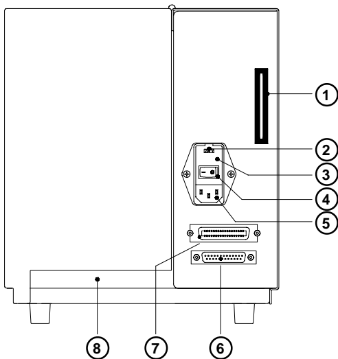
Bild 4 f Rückansicht Apollo 1/2
