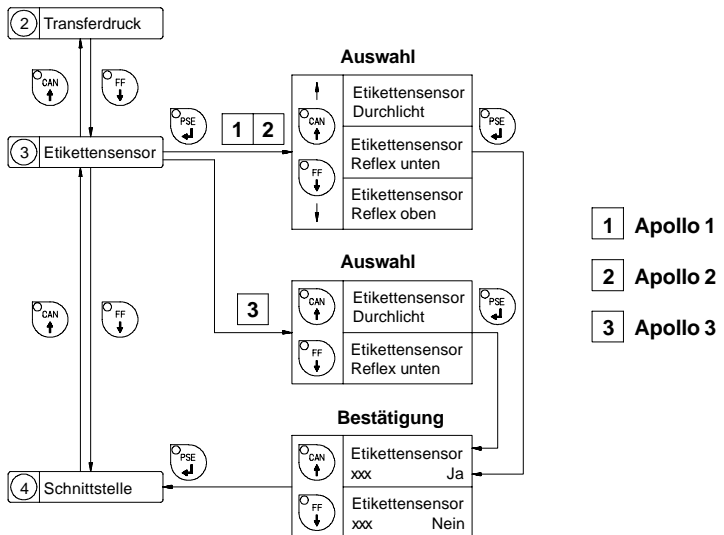
Bild 9 d Einstellung des Parameters "Etikettensensor"
