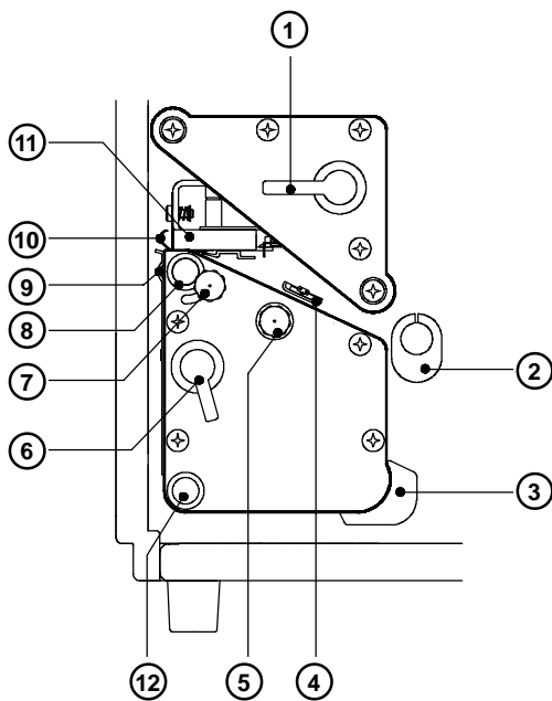
Bild 4 e Detailansicht Druckmechanik Apollo 2/3
