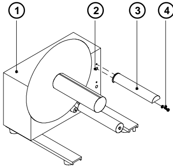
Bild 13 c Montage der Umlenkung
