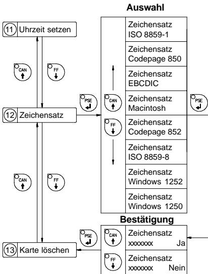
Bild 9 n Einstellung des Parameters "Zeichensatz"
