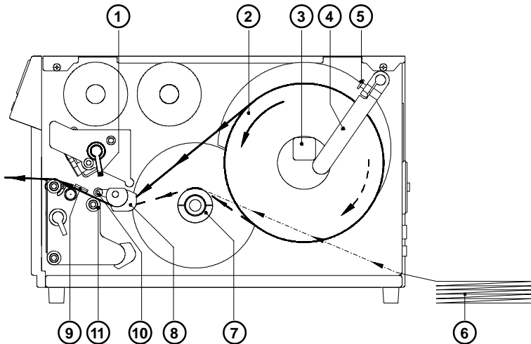
Bild 6 a Einlegen der Etiketten Apollo 1
