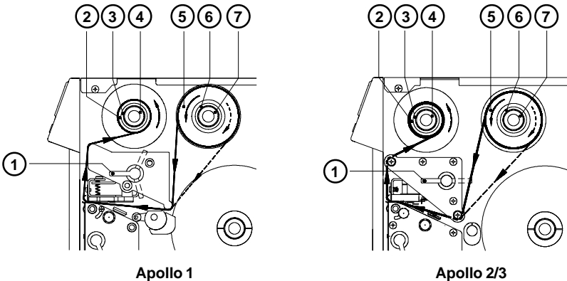
Bild 6 c Einlegen des Transferbandes
