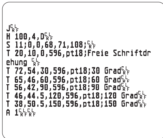
Bild 12 b Ausdruck des Beispieltickets im Monitormodus
