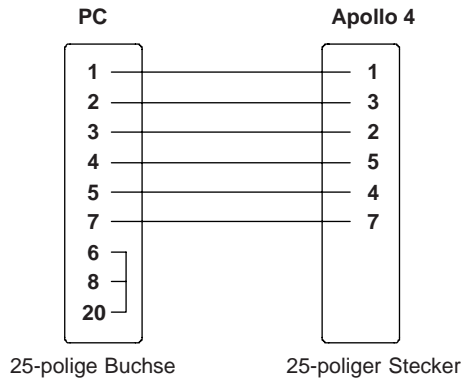
Bild B-4 Schnittstellenkabel mit 25-poligem Computeranschluß für RS-232 mit Protokoll "RTS/CTS" bzw. "XON/XOFF"
