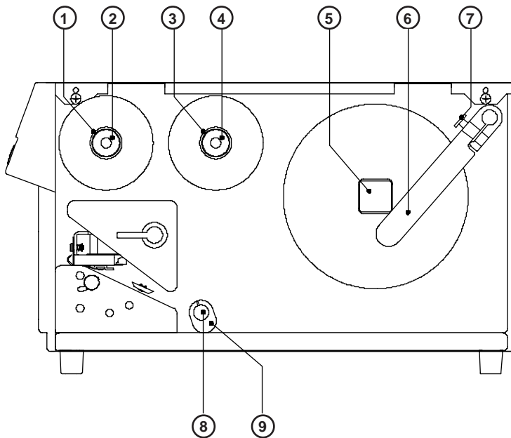
Bild4 b Seitenansicht (bei offenem Deckel)
