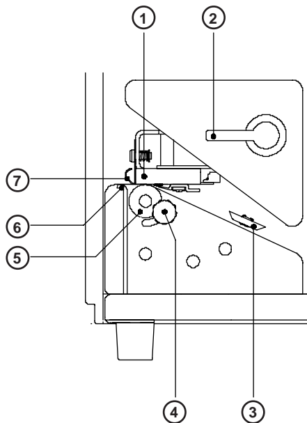
Bild 4c Detailsicht Druckmechanik
