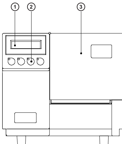
Bild 4 a Frontansicht
