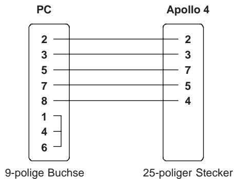
Bild B-5 Schnittstellenkabel mit 9-poligem Computeranschluß für RS-232 mit Protokoll "RTS/CTS" bzw. "XON/XOFF"
