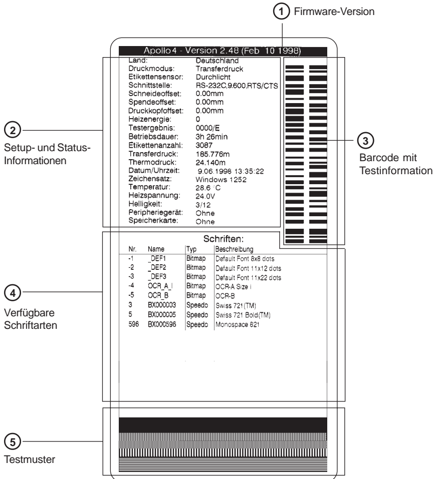
Bild 10 Selbsttestausdruck
