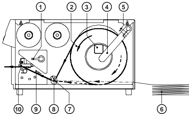
Bild 6 a Einlegen der Etiketten
