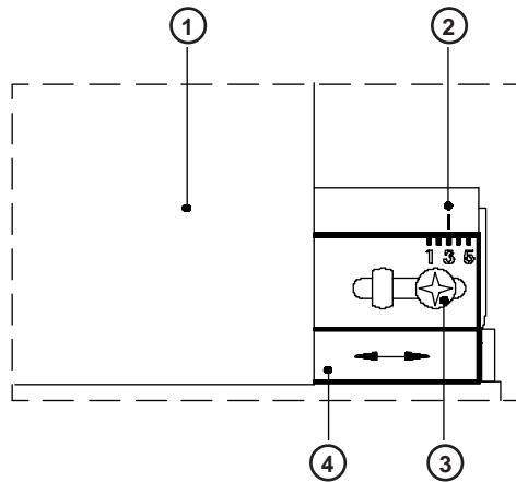
Bild 7b Justage des Transferbandlaufes
