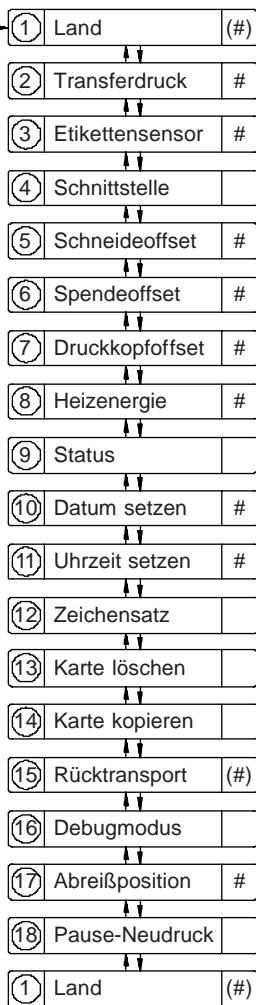
Bild 9 a Setup-Parameter
