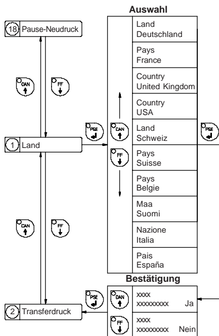
Bild 9 b Einstellung des Parameters "Land"
